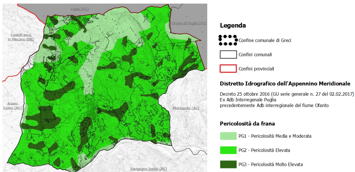
Figura 23 – Stralcio della tavola di pericolosità da frana del PdP.
