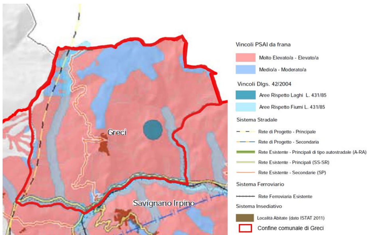
Figura 21 – Greci nella Fig.3 dell'elaborato "P.11.16 Città dell'Arianese" del Ptcp di Avellino – Rischi e vincoli
