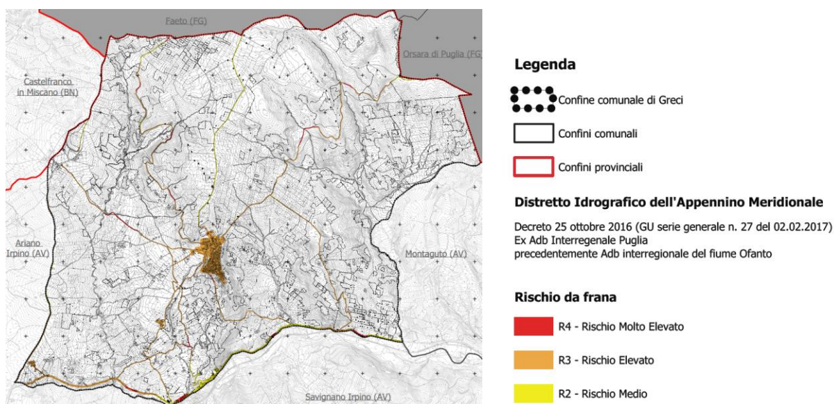
Figura 24 - Stralcio della tavola del rischio da frana del PdP.
