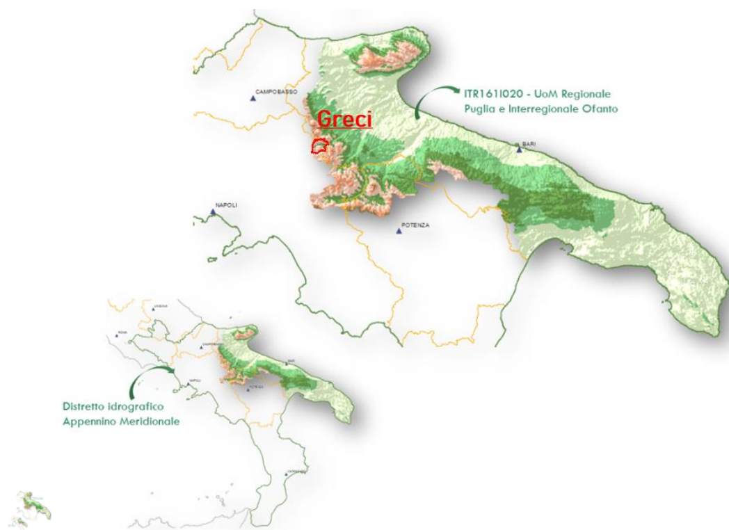
Figura 22 – Greci nella perimetrazione dell’UoM Regionale Puglia e interregionale Ofanto confluyente nell’ ex Autorità di Bacino Interregionale Puglia, poi confluito nel Distretto idrografico Appennino Meridionale
