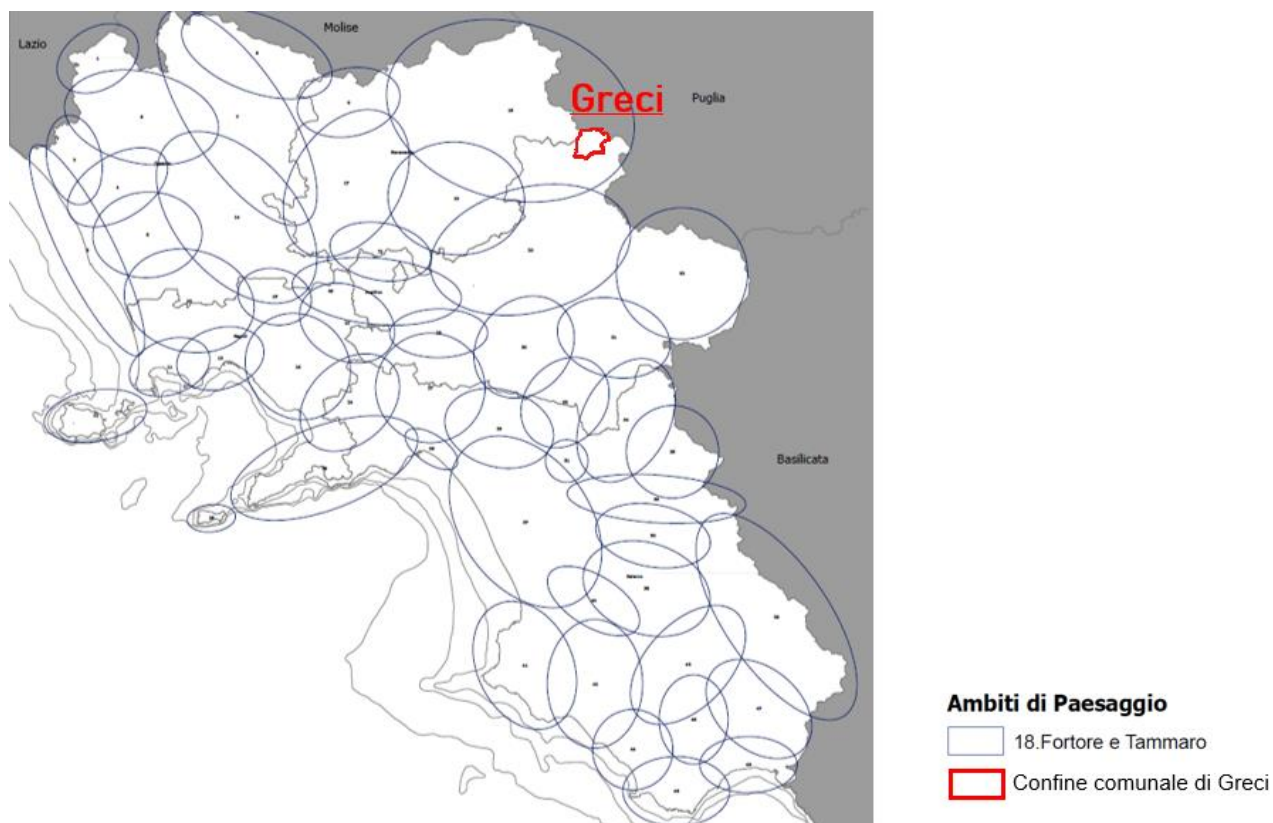
Figura 13 – Greci nelle Linee guida per il paesaggio: gli ambiti di paesaggio
